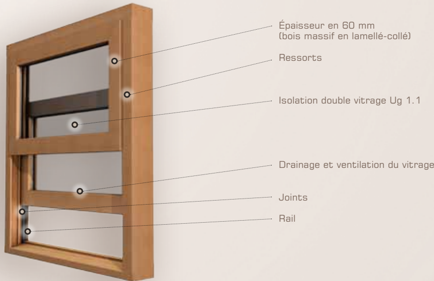
Le châssis guillotine à ressorts
